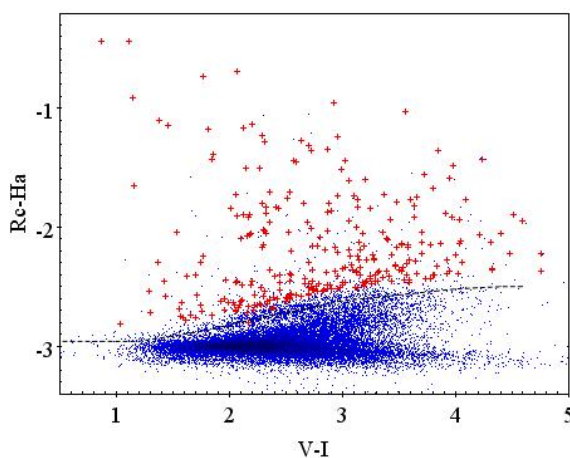
Рис.1. Диаграмма зависимости меры эмиссии ( R - H\alpha ) и показателя цвета ( V-I ).
