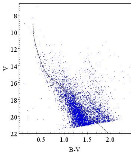
Рис. 4. Диаграмма показатель цвета – звездная величина ( V, B-V ) IC 1848.
