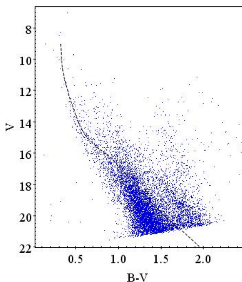
4 – расм. IC 1848 нинг ранг кўрсаткичи – юлдуз катталиги диаграммаси.
