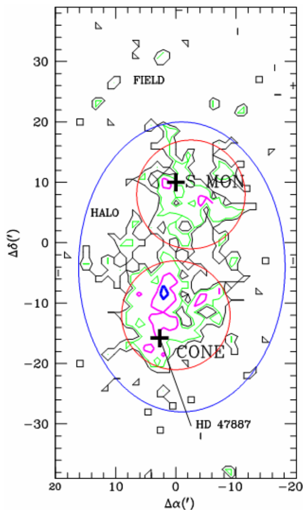
Рис. 2. Карта поверхностной плотности звезд, показывающих H\alpha эмиссию.
