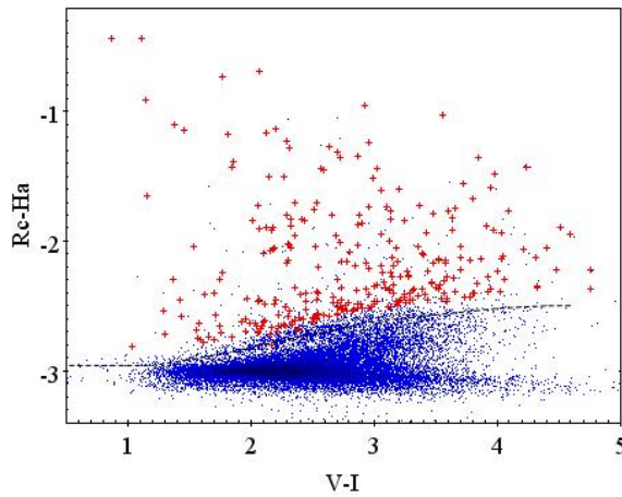
1 – расм. ( R-H\alpha ) эмиссия ўлчовини ( V-I ) ранг кўрсаткичига боғлиқлиги диаграммаси.
