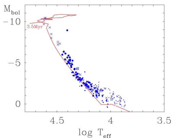
Рис. 5. Диаграмма Герцшпрунга-Рассела IC 1805.
