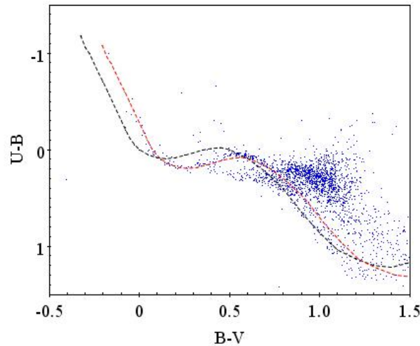
Рис. 3. Двухцветная диаграмма NGC 2353.
