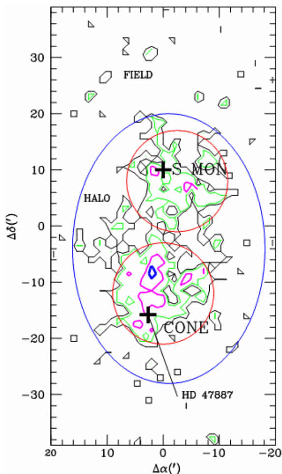
2 – расм. На эмиссиясини намоён қилувчи юлдуздарнинг юза зичлиги харитаси.
