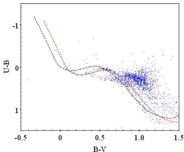
3 – расм. NGC 2353 нинг икки рангли диаграммаси.
