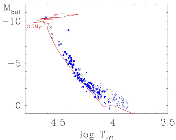
5 – расм. IC 1805 нинг Герцшпрунг – Рассел диаграммаси.
